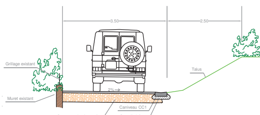
Coupe-type C-C'
