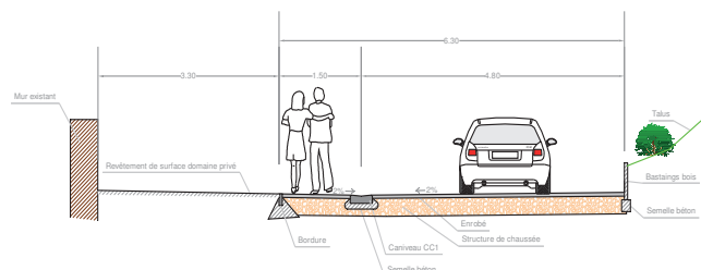
Coupe-type A-A'
